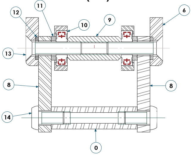
A-A (1 : 1)
