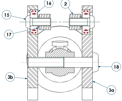
B-B (1 : 1)
