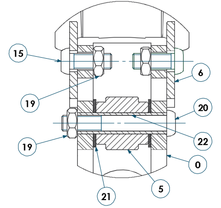
D-D (1 : 1)
