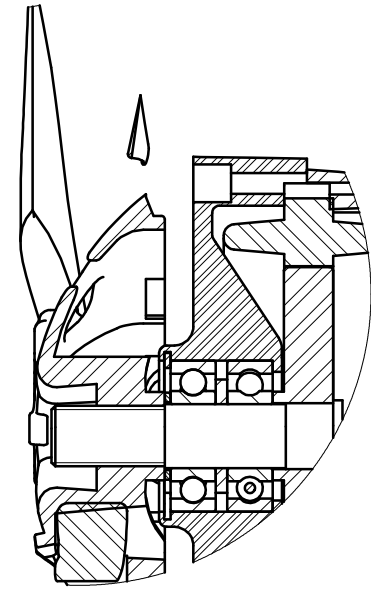
DÉTAIL B ECHELLE 1 : 2
